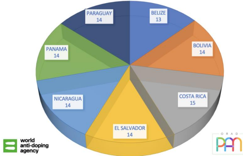
Gráfica 1: Muestra la cantidad de controles y porcentajes realizados por cada país según su cuota de la beca de WADA 2024. Costa Rica realizó un total de 15 controles. Los países que realizaron un total de 14 controles fueron: Paraguay, Panamá, Nicaragua, El Salvador y Bolivia. El país que realizó 13 controles fue: Belice.
