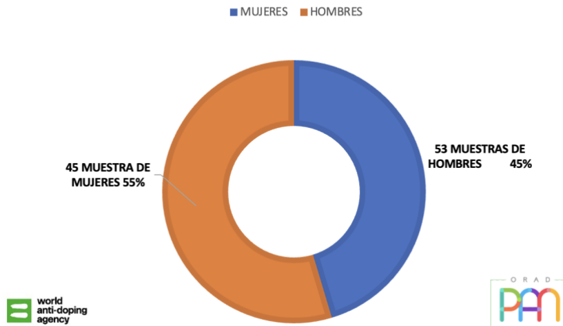
Gráfica 2: Controles realizados por sexo según la beca 2024. Un total de 55% de muestras realizadas a mujeres (45) y un 45% realizadas a hombres (53).
