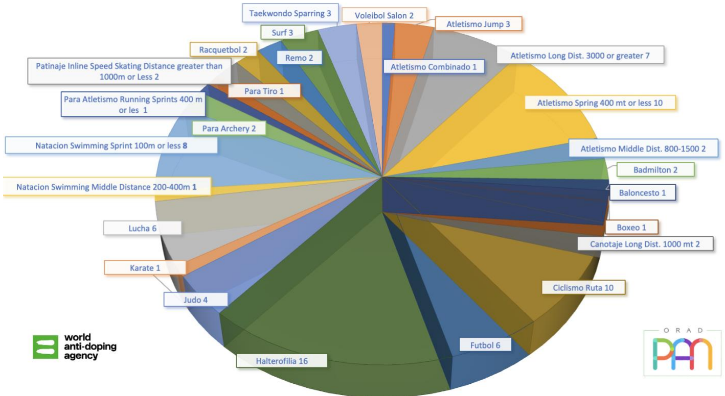
Gráfica 3: Controles realizados por deporte. Destacando Atletismo larga distancia con un total de 7 controles, Natación con 8 controles, Ciclismo de Ruta con 10 controles y Culturismo con 16 controles como los deportes en los cuales se realizó mayor cantidad de muestras.
